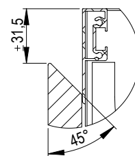
DETTAGLIO C SCALA 1:2
