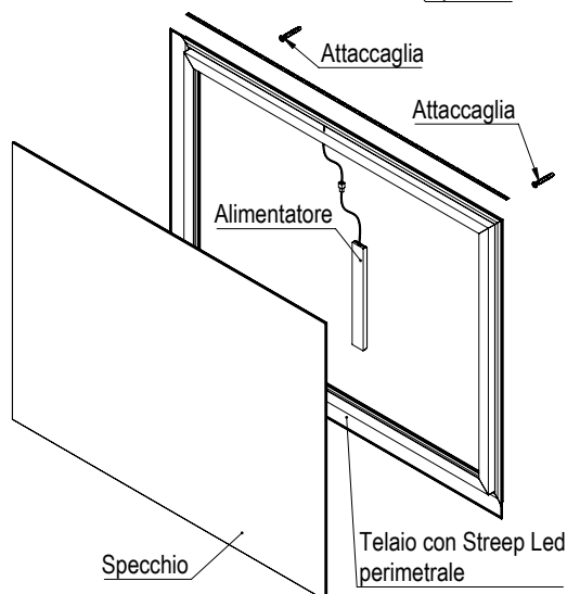
SEZIONE A-A
